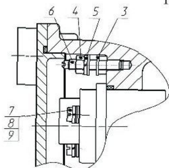
Рисунок 2 – Сборка внутреннего заземления
