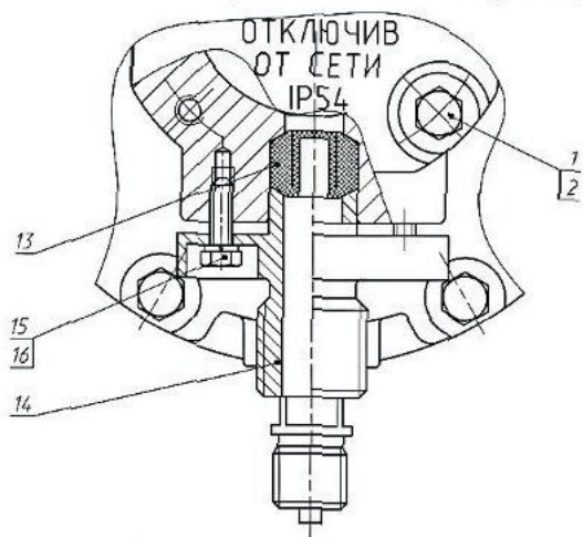
Рисунок 1 – Сборка фланца
