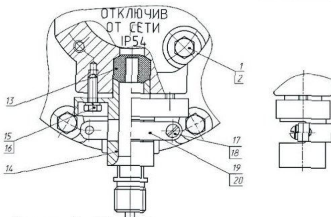
Рисунок 4 – Сборка фланца для первого варианта
